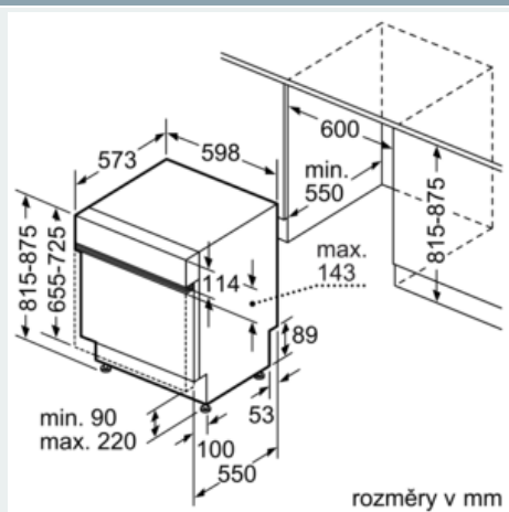
Rozměrové výkresy
